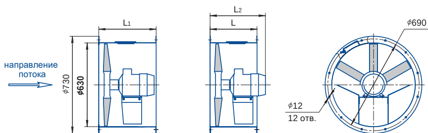
тип корпуса 01
