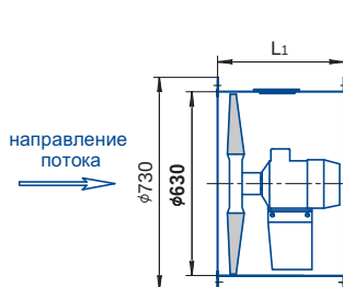
тип корпуса 01
