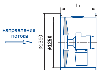
тип корпуса 01
