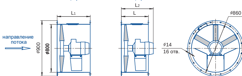
тип корпуса 01
