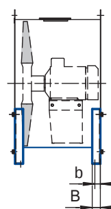
Вентилятор серии ОСА
