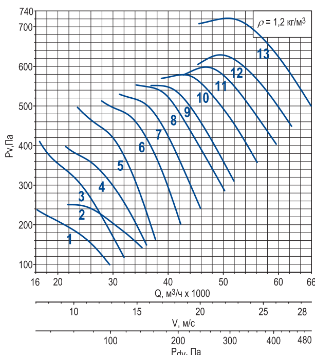
тип корпуса 01
