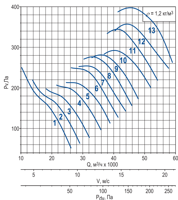
тип корпуса 02
