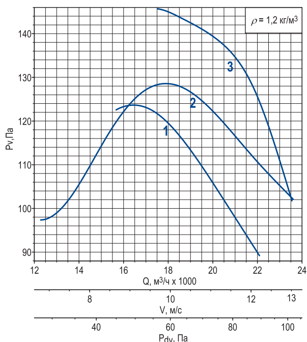
тип корпуса 01
