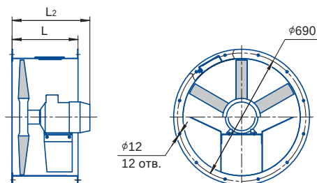
тип корпуса 02
