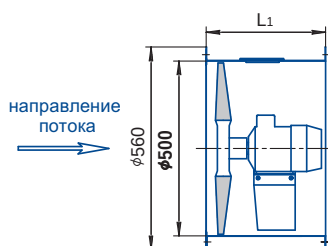
тип корпуса 01
