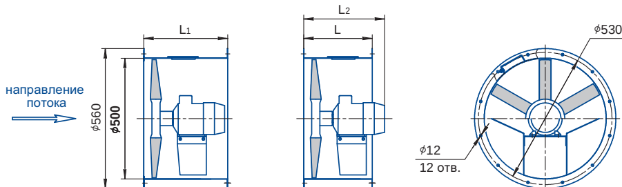
тип корпуса 01
