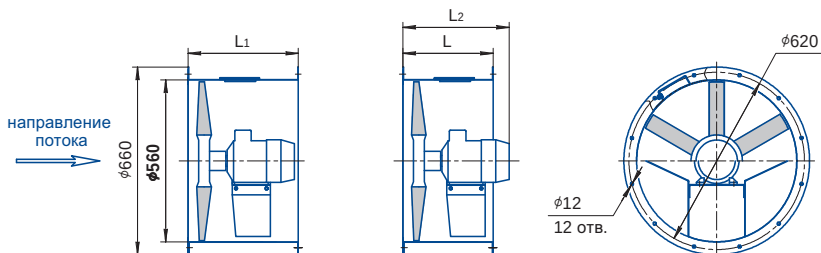
тип корпуса 01
