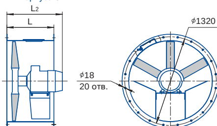
тип корпуса 02
