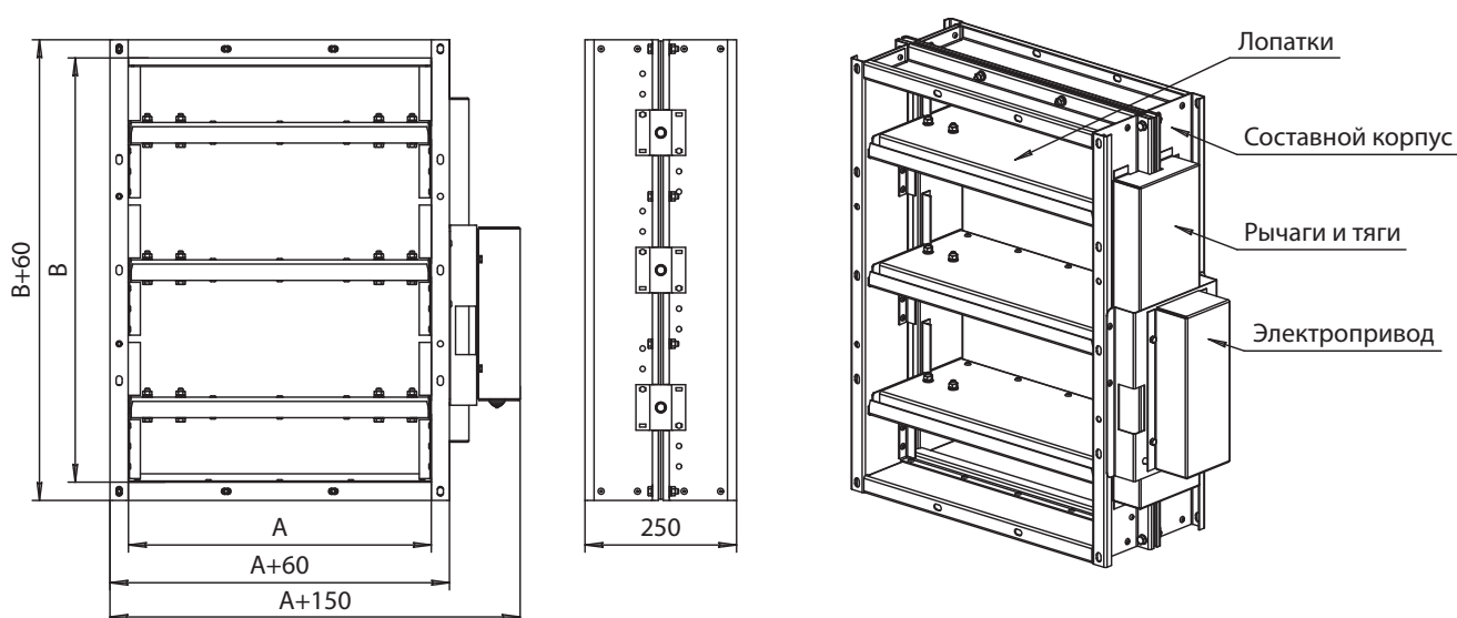
Противопожарный клапан НЕРПА-КП общего назначения
