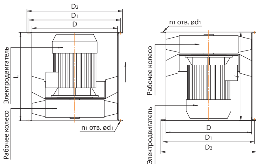
Вентилятор судовой ОС вертикальный без опоры с рабочим колесом вверху или внизу (с направлением потока вверх или вниз)
