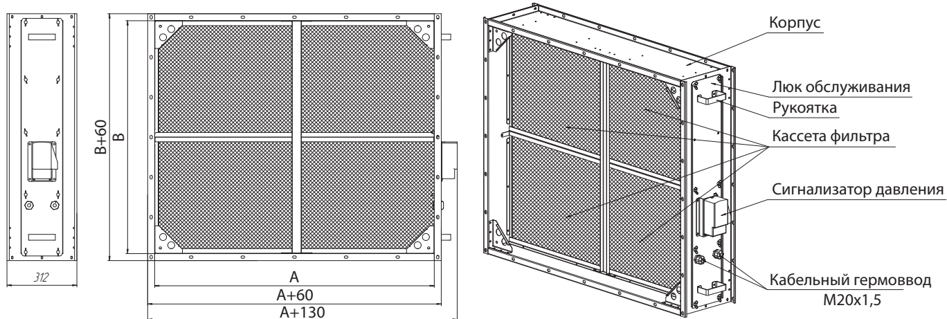
Воздушный фильтр ФКМ с одной стороной обслуживания справа (П) или слева (Л)
