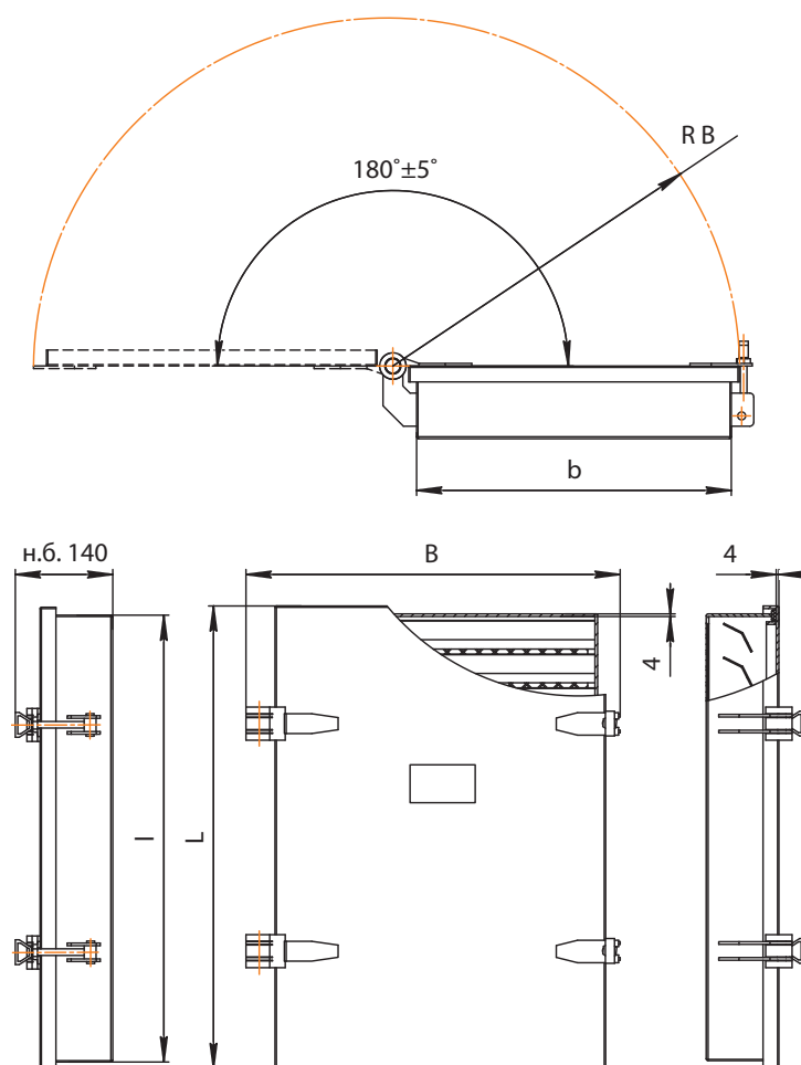
Односекционная водогазонепроницаемая крышка НЕВА
